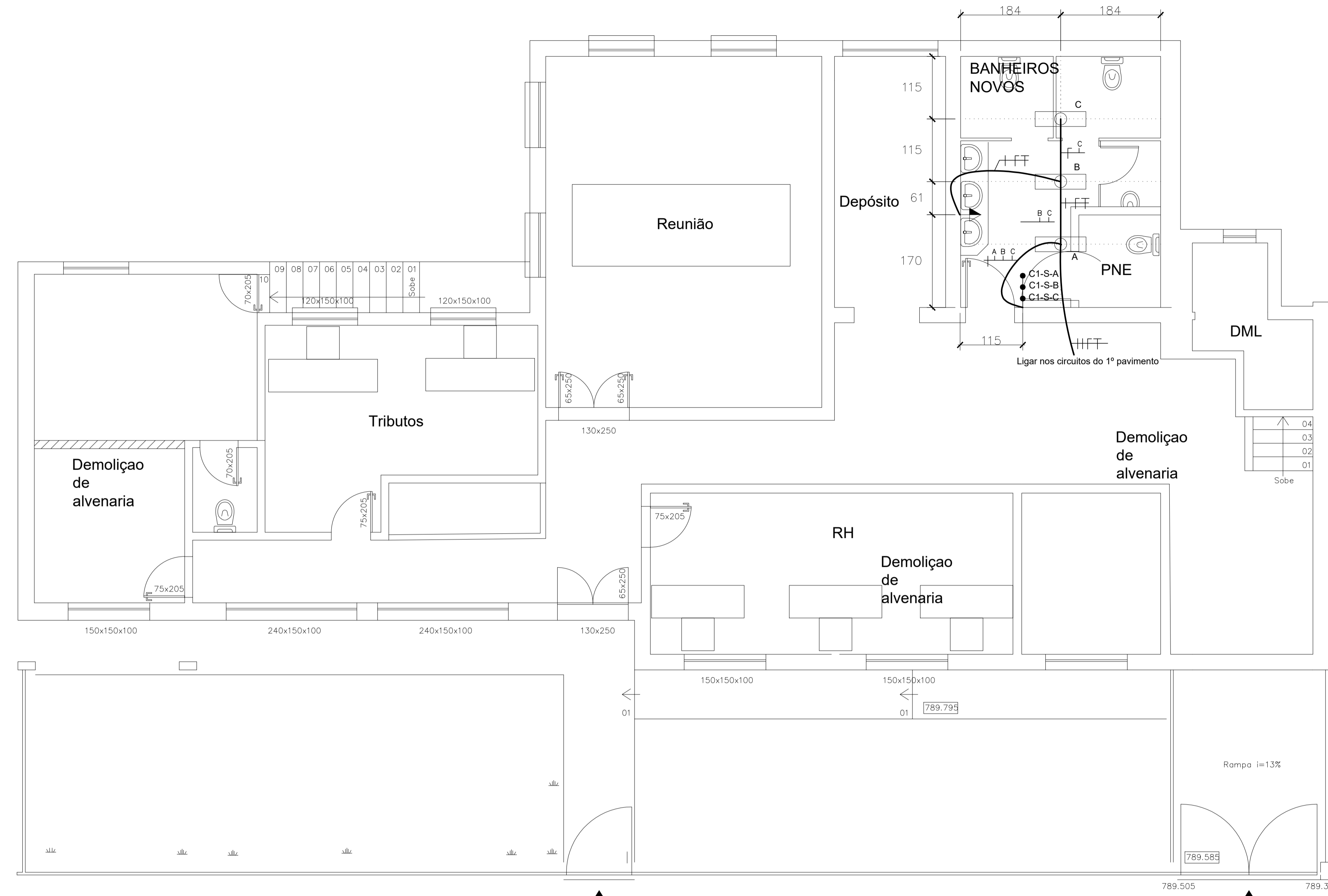
PLANTA BAIXA DO 1º PAVIMENTO Escala 1:50
