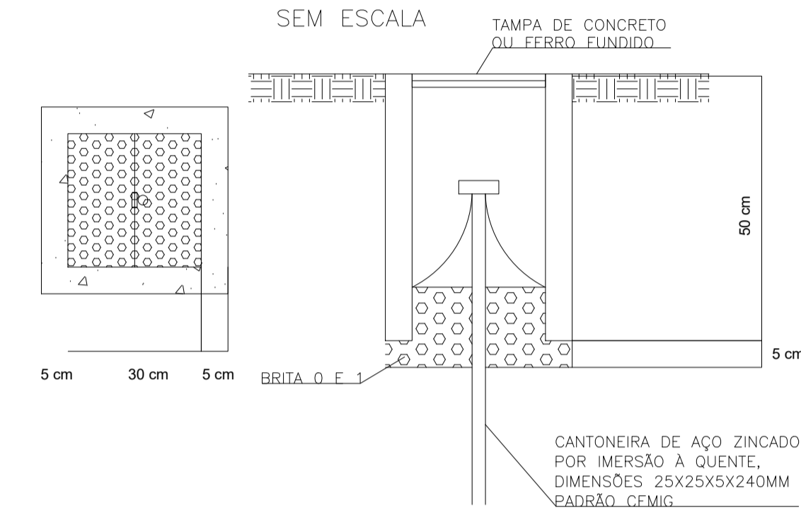
DETALHE DA CAIXA DE INSPEÇÃO SEM ESCALA
